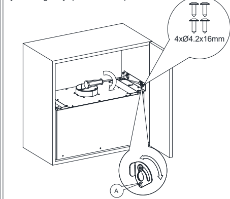
Rys. 8. Regulacja położenia okapu.
