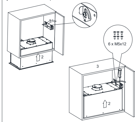
Rys. 7b. Montaż okapu.
