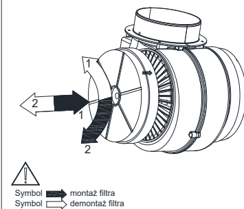
Rys. 9 Wymiana filtra węglowego.
