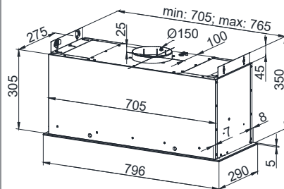
Rys. 2 Rysunek gabarytowy.
