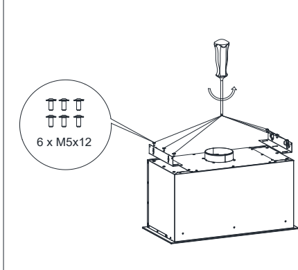
Rys. 6 Demontaż kątowników montażowych.
