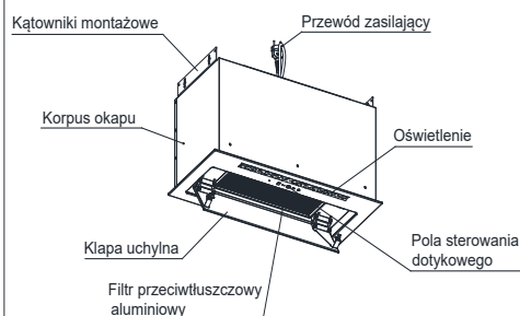
Rys.1 Rysunek poglądowy okapu kuchennego
