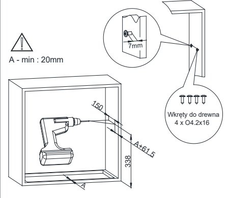
Rys. 7a Montaż okapu.
